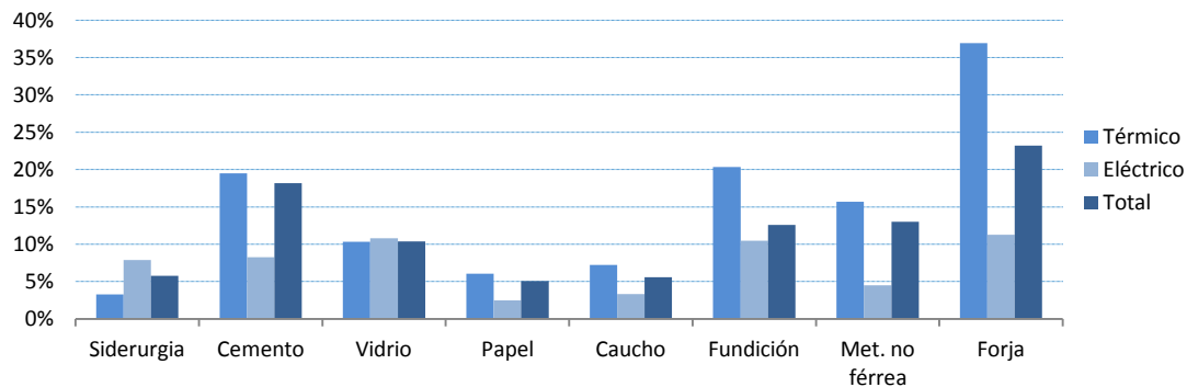
Figura 40. Potenciales técnicos de ahorro energético en sectores industriales grandes consumidores vascos. (Fuente: EVE)
