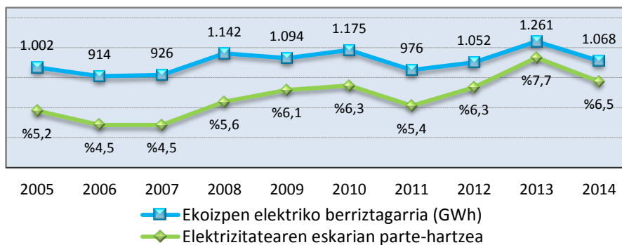
54. irudia. Ekoizpen elektrikoaren bilakaera Euskadin eta eskari elektrikoan duen parte-hartzea, 2005-2014. (Iturria: EEE)
