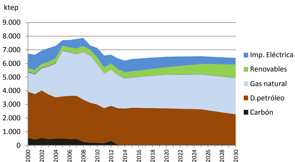
Figura 26. Euskadi. Demanda energética 2030. Escenario de Políticas Energéticas (Fuente: EVE)
