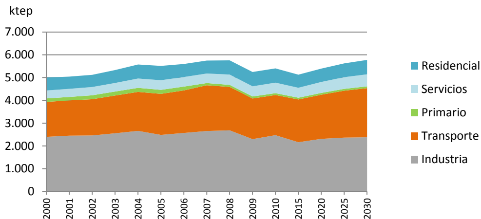
Figura 23. Euskadi. Consumo energético sectorial 2015-2030. Escenario tendencial (Fuente: EVE)
