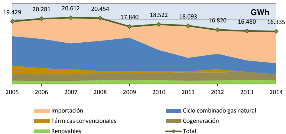
Figura 6. Consumo total y fuentes de abastecimiento de energía eléctrica en Euskadi (Fuente: EVE)
