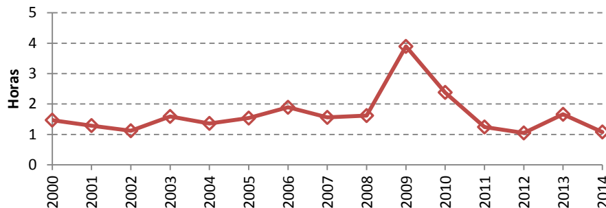
Figura 59. Evolución del TIEPI en Euskadi
