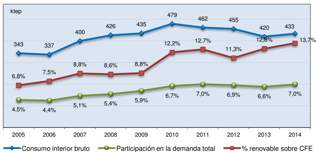
Figura 10. Evolución del aprovechamiento de las energías renovables en Euskadi y participación de las renovables en la demanda total de energía y en el consumo final de energía (CFE) (Fuente: EVE). Nota: La cuota de renovables sobre consumo final de energía (CFE) incluye la energía eléctrica renovable importada.
