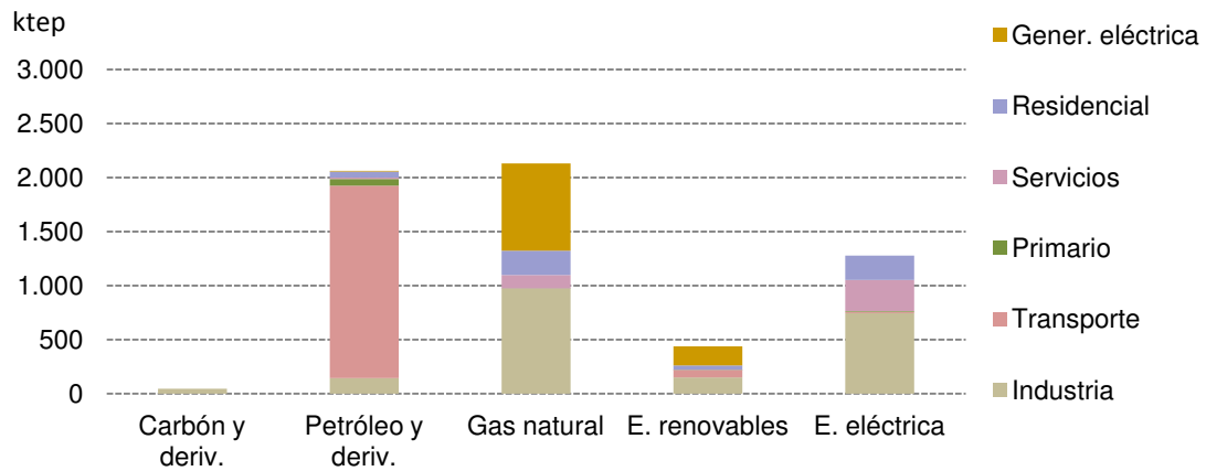
Figura 3. Reparto por sectores para cada tipo de energía, año 2014 (Fuente: EVE)
