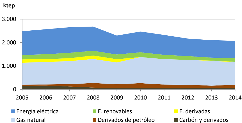
Figura 36. Evolución del consumo industrial de energía en Euskadi (Fuente: EVE)
