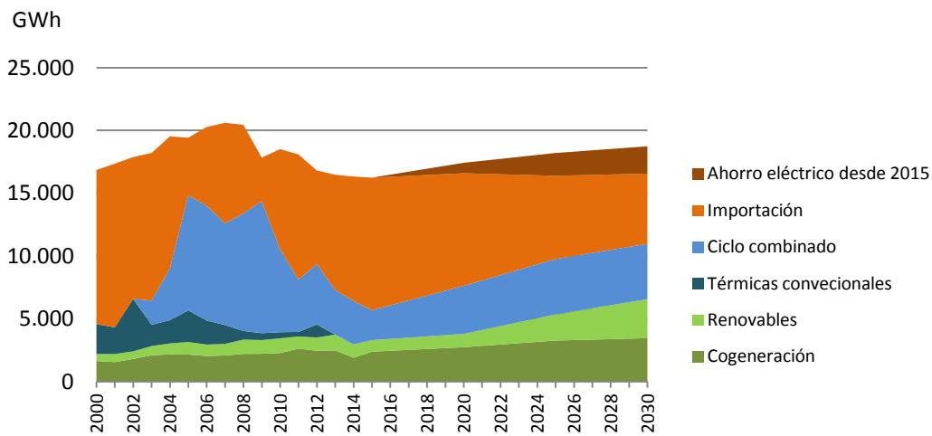
Figura 29. Euskadi. Suministro eléctrico 2030. Escenario de Políticas Energéticas (Fuente: EVE)
