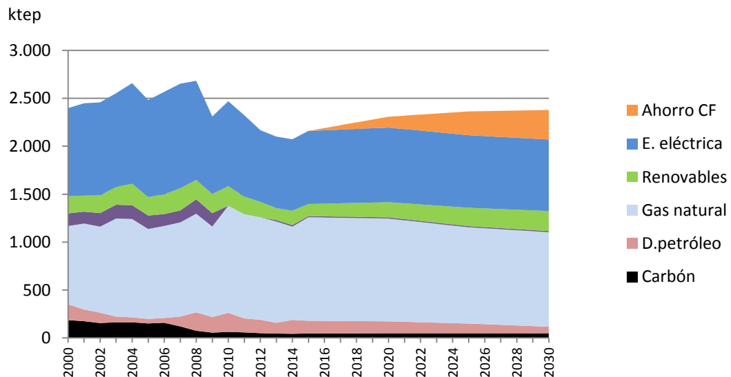
Figura 42. Escenario de consumo energético industrial (Fuente EVE)
