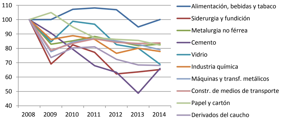
Figura 38. Evolución del consumo eléctrico 2008-2014 por subsectores industriales en Euskadi (índice 2008=100) (Fuente: EVE, basado en datos de Iberdrola)
