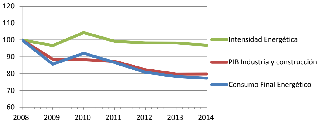
Figura 37. Evolución de la intensidad energética en la industria en Euskadi en términos de consumo de energía por unidad de PIB (índice 2008=100) (Fuente: EVE)
