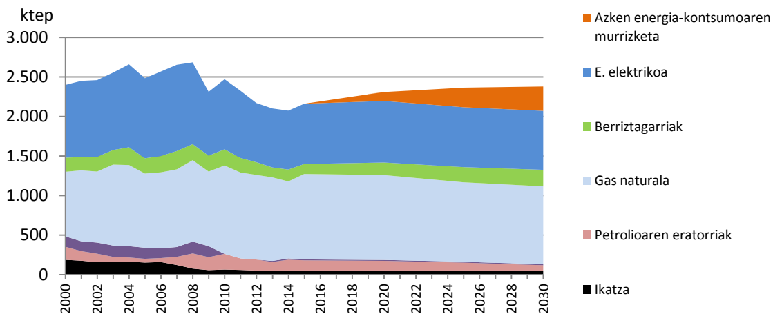
42. irudia. Industriako energia-kontsumoaren egoera garraioan. (Iturria: EEE)
