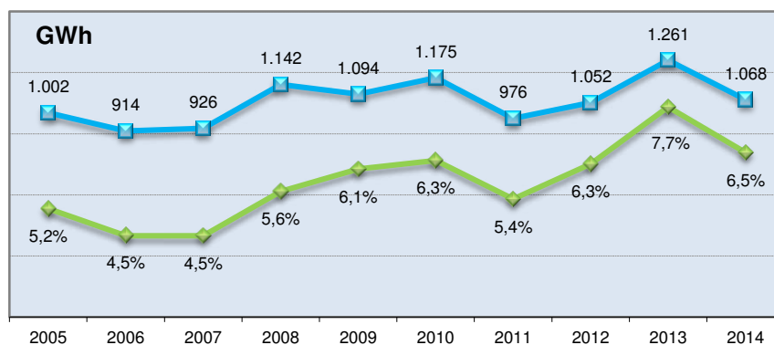
Figura 8. Evolución de la producción eléctrica renovable en Euskadi, en valores absolutos (GWh) y relativos (% sobre la demanda eléctrica total) (Fuente: EVE)
