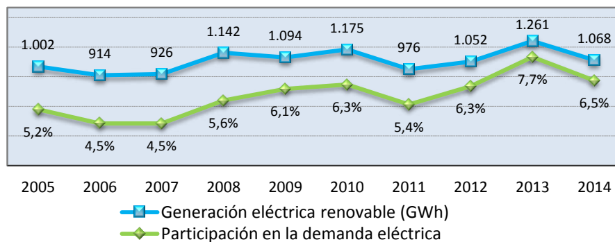
Figura 54. Evolución de la producción eléctrica en Euskadi y su participación en la demanda eléctrica, 2005-2014. (Fuente: EVE)
